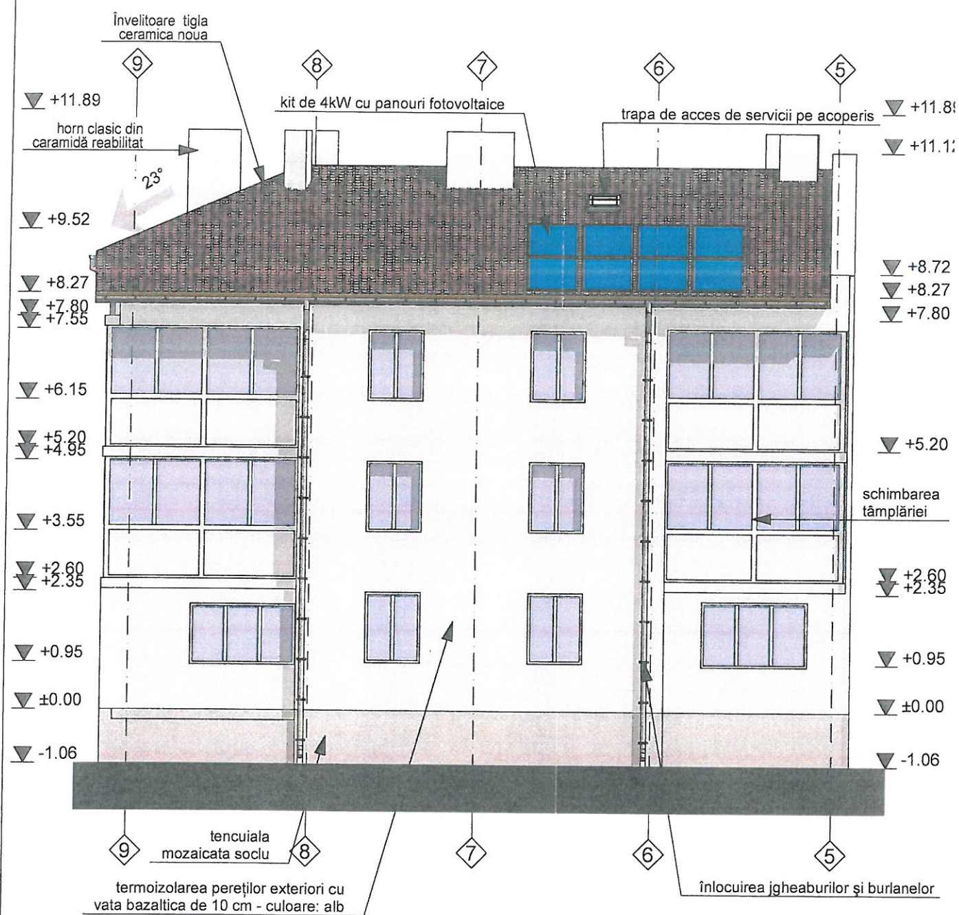
FAȚADĂ PRINCIPALĂ BLOC 4 PROPUȘ
