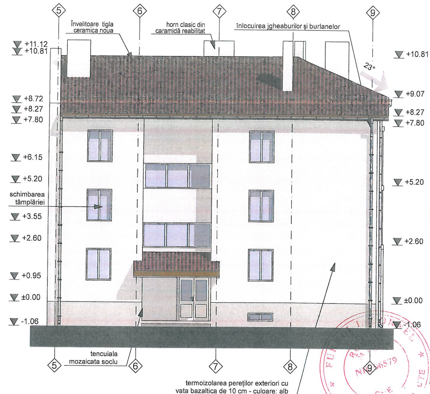
FAȚADĂ SECUNDARĂ BLOC 4 PROPUȘ
