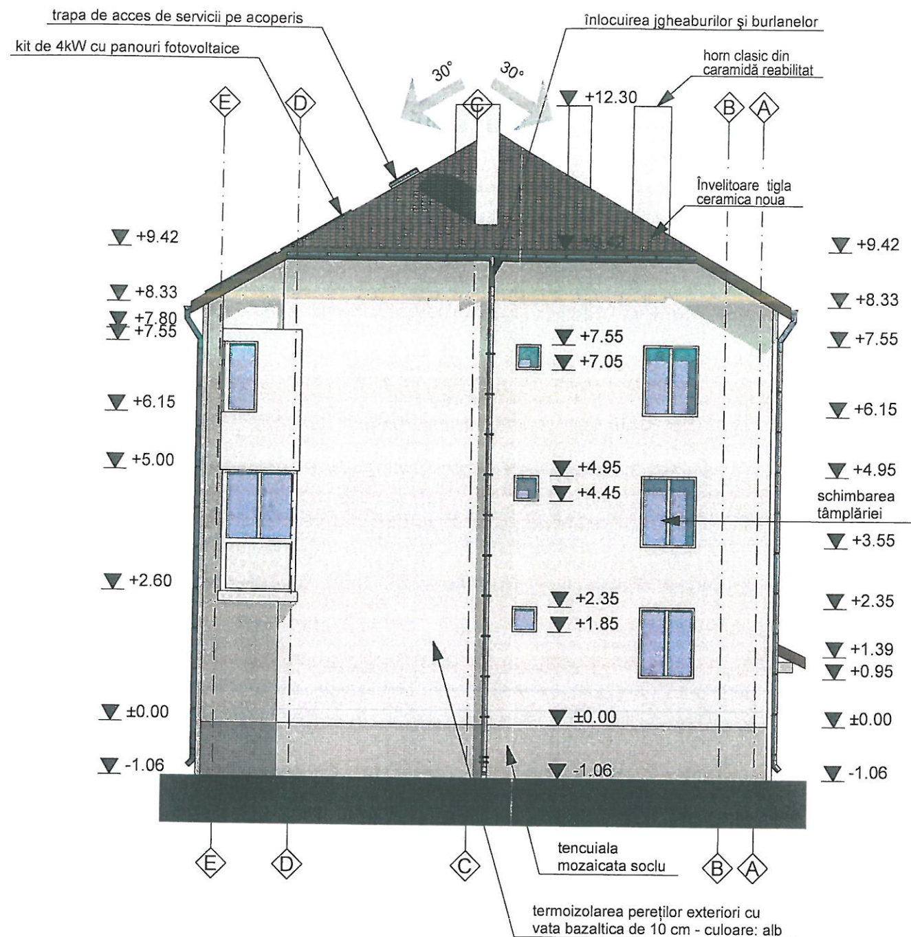
FAȚADĂ DREAPTĂ BLOC 1 PROPUS
