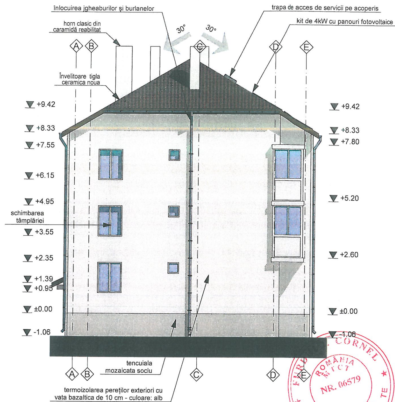
FAȚADĂ STANGĂ BLOC 1 PROPUS
